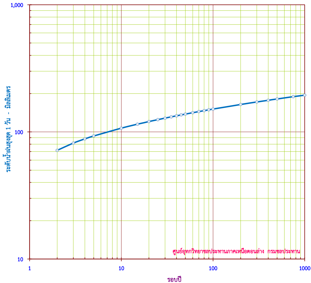
กราฟแสดง ปริมาณน้ำฝนสูงสุด1วัน ขนาดรอบปีต่างๆ สถานี 630181 อ.แม่สอด จ.ตาก
